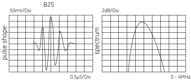
0.5 µ S/Div 0 - 4MHz 典型波形和频谱
