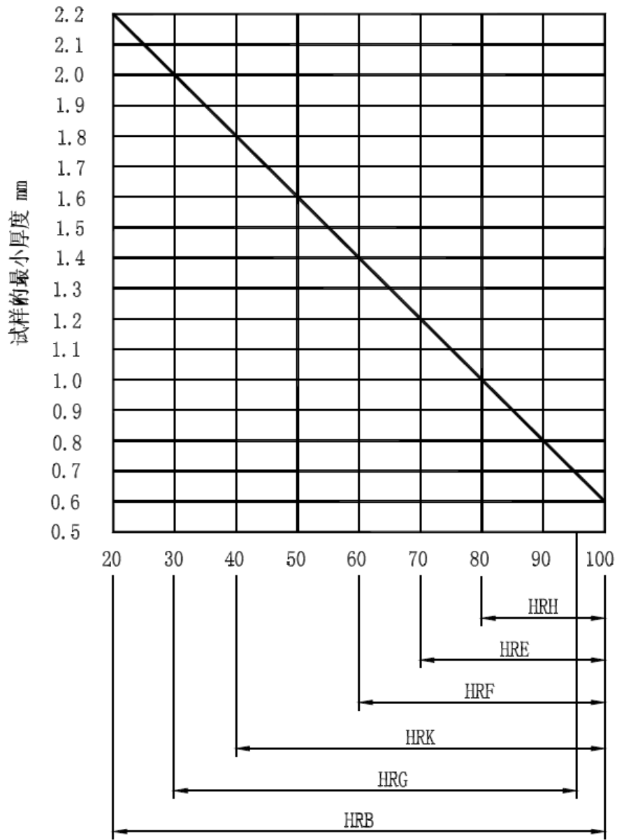
附图 3 用钢球压头试验 (HRB、HRE、HRF、HRG、HRH、HRK)
